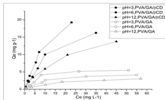
Figure 4. Equilibre d'adsorption de 2-chlorophénol sur les membranes PVA/GA/ \beta -CD et PVA/GA à différents \text{pH} (3, 6, 12) ( T=294\text{K} , 8% \beta -CD, 100mg/L).
