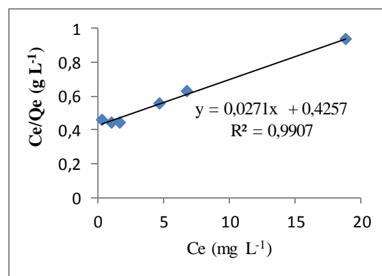
Figure 5. Adaptation linéaire au modèle de Langmuir des données d'adsorption du 2-chlorophénol sur la membrane polymère PVA / GA / \beta -cyclodextrine à \text{pH} = 3
