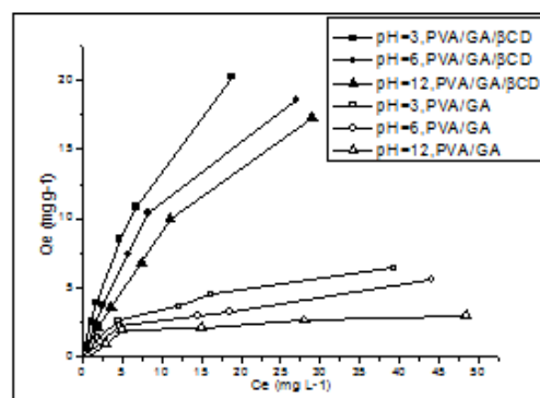
Figure 2. Equilibre d'adsorption de 2-chlorophenol sur les membranes PVA/GA/ \beta -CD et PVA/GA à différents pH (3, 6, 12) ( T=294\text{K} , 8% \beta -CD, 100\text{mg/L} ).
