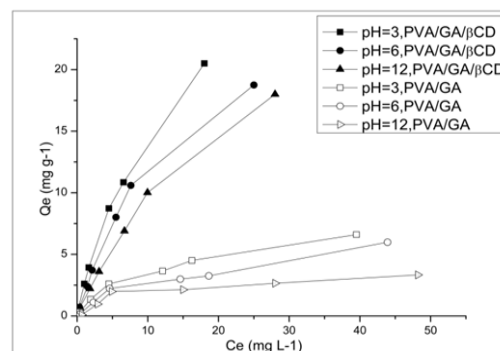
Figure 3. Equilibre d'adsorption de 2-Nitrophenol sur les membranes PVA/GA/ \beta -CD et PVA/GA à différents pH (3, 6, 12) ( T=294\text{K} , 8% \beta -CD, 100\text{mg/L} ).
