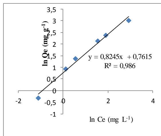
Figure 6. Adaptation linéaire au modèle de Freundlich des données d'adsorption du 2-chlorophénol sur la membrane polymère PVA / GA / \beta -cyclodextrine à \text{pH} = 3 .
